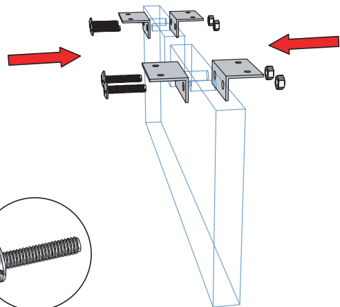
M6x30
